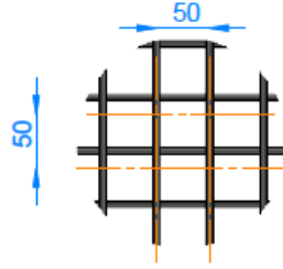
DETAY F ÖLÇEK 1 : 5
